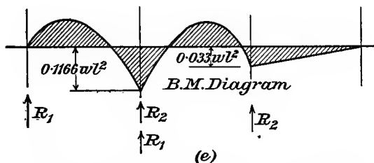
FIG. 65 (d) and (e).—Three spans, one bay unloaded.
